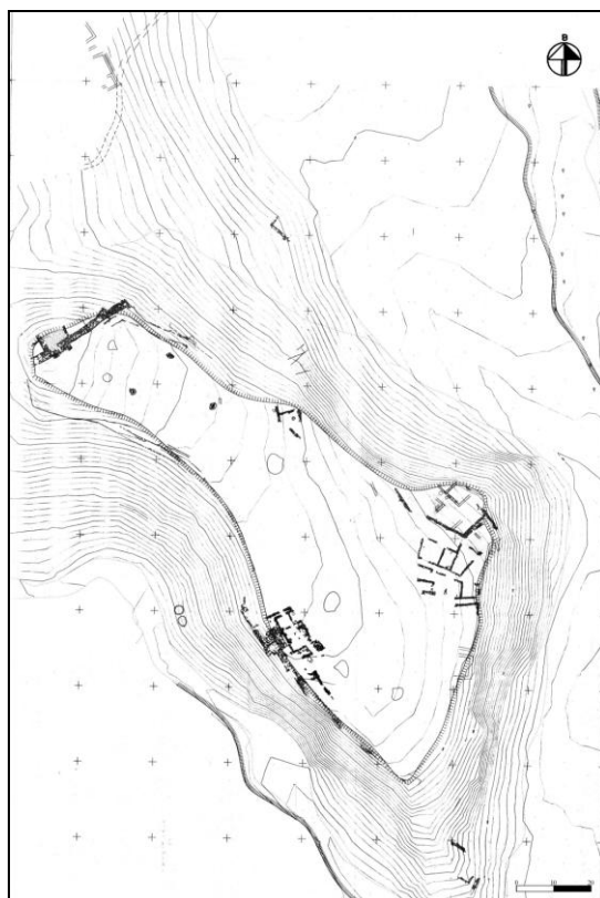
Σχ.1: Τοπογραφικό διάγραμμα της ακρόπολης των Λειβήθρων
